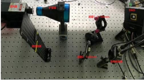
单像素成像实验光路图
