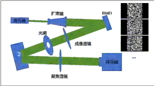
单像素成像系统示意图
