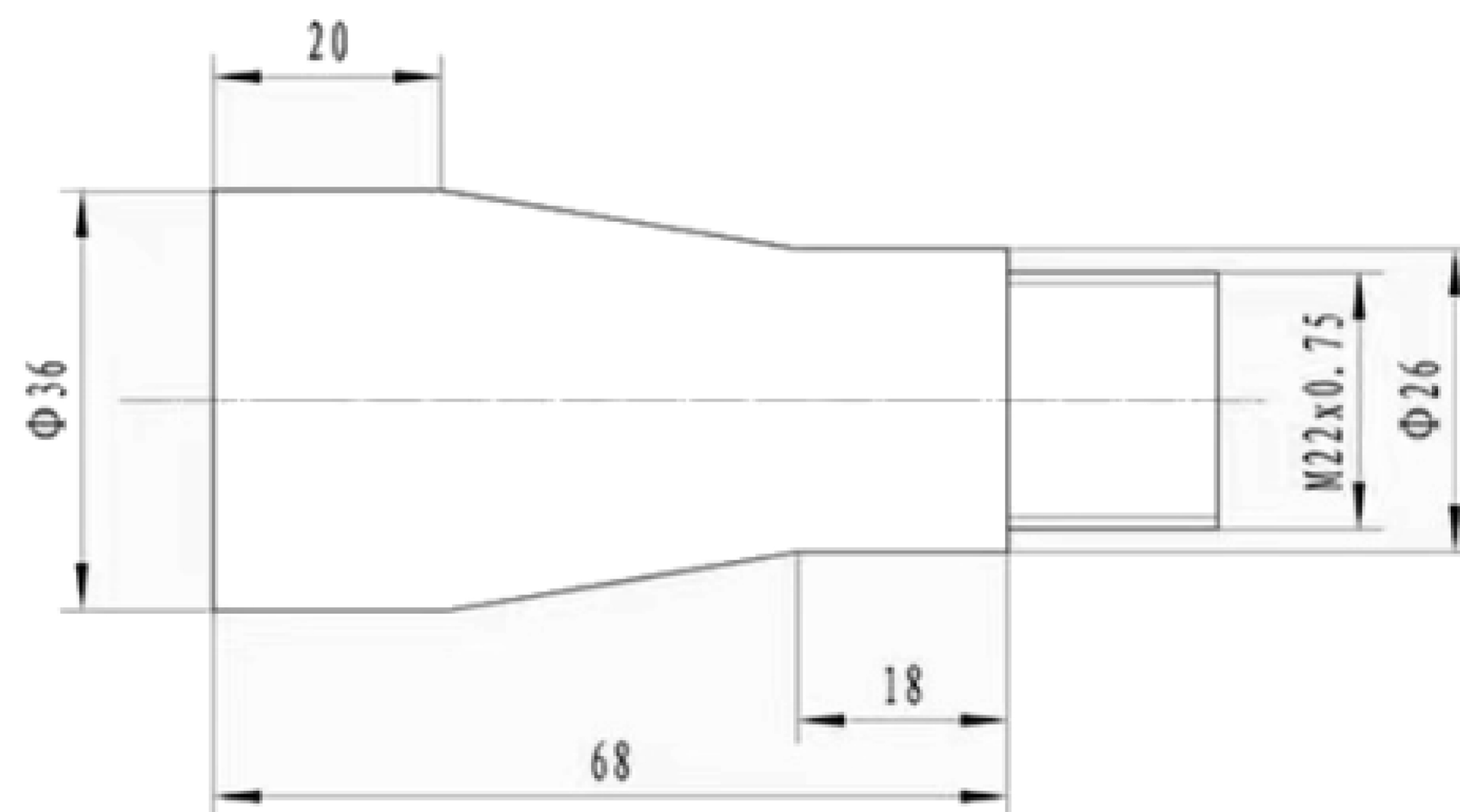
6倍扩束镜
